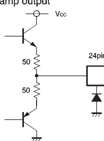
Op-amp output
