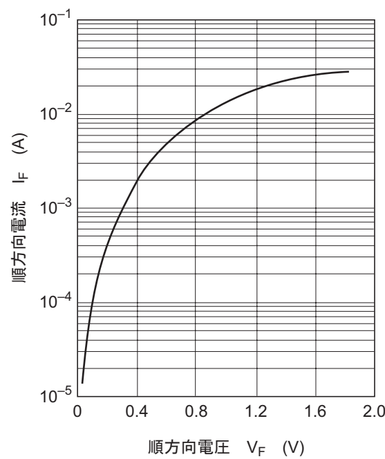
图1. 順方向特性
