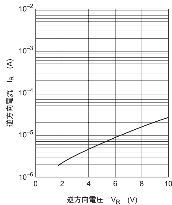
图2. 逆方向特性
